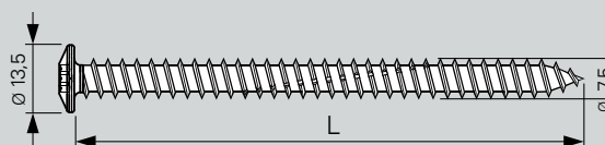
FB-FK talířová hlava, Torx 30
